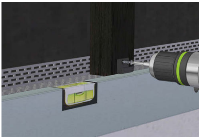
Montage Startklammer
