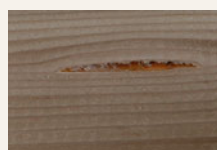
Weiche oder harte Harzaus- tritte (Harzgallen/-taschen)
