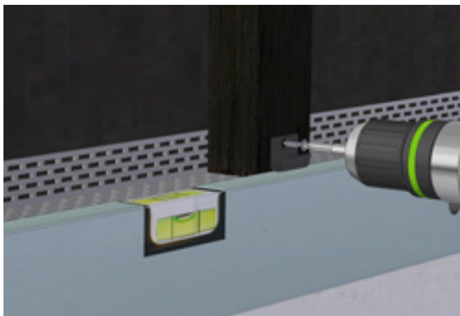
Montage Startklammer
