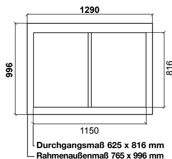
Detail-Zeichnung Doppelfenster Alina
