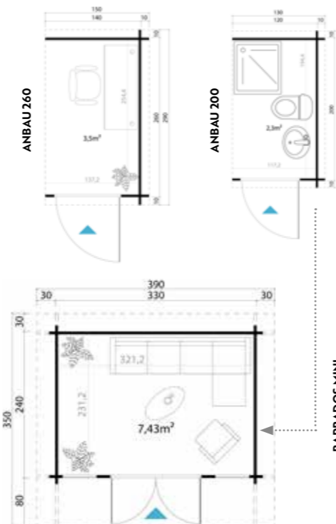
Passend für Gartenhäuser ab einer Wandtiefe von 200 cm. Ideal als Abstellraum – perfekt geeignet für unsere Barbados-Serie oder andere Pultdachmodelle
