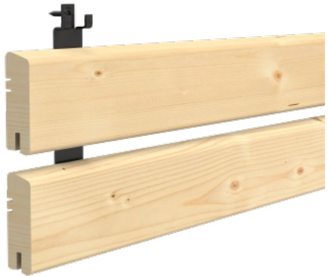
Verdeckte Befestigung mit solider, schwarzer Fassadenklammer
